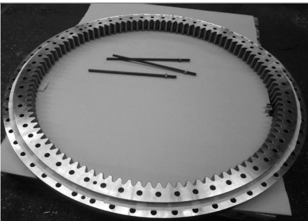
Okretni ležaj gondole
