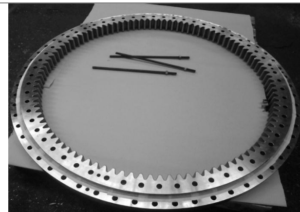
Okretni ležaj gondole
